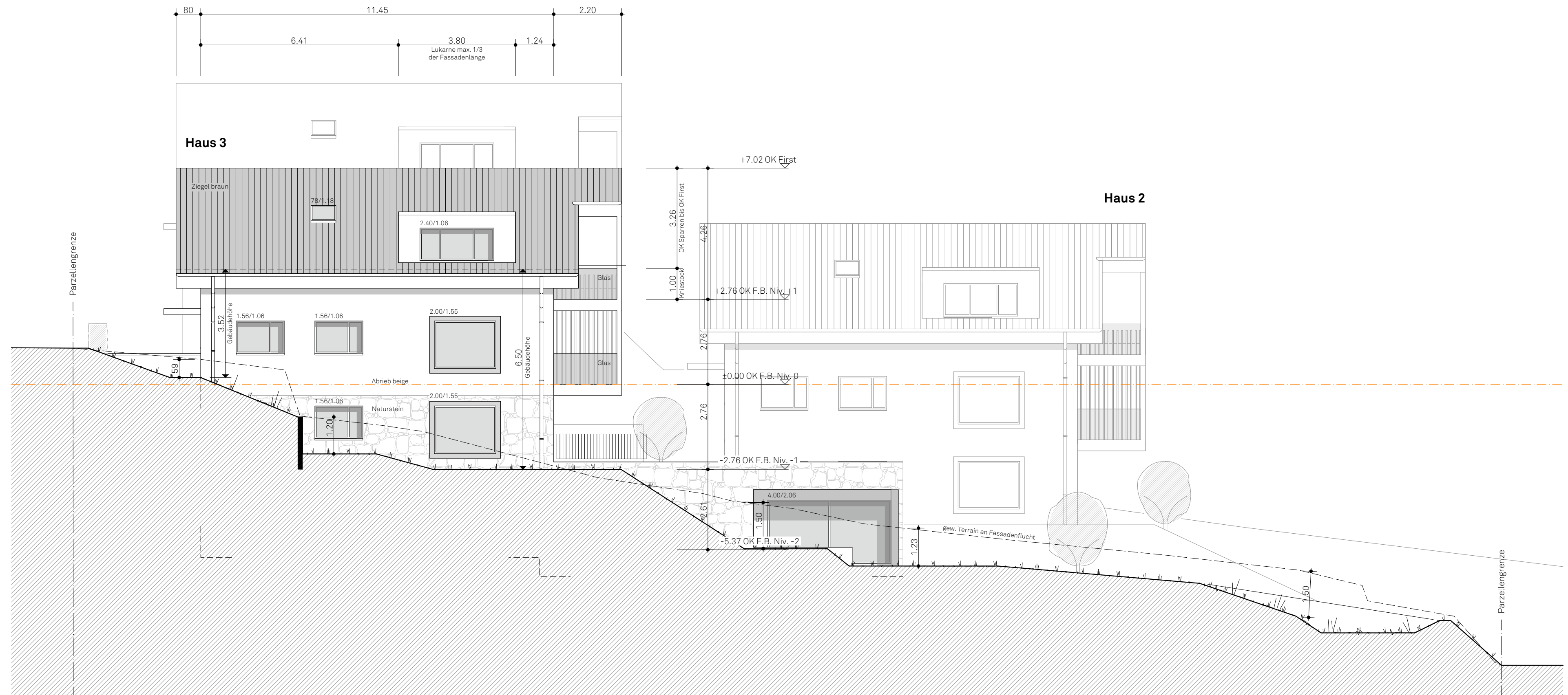
Haus 3 - Nordwestfassade
