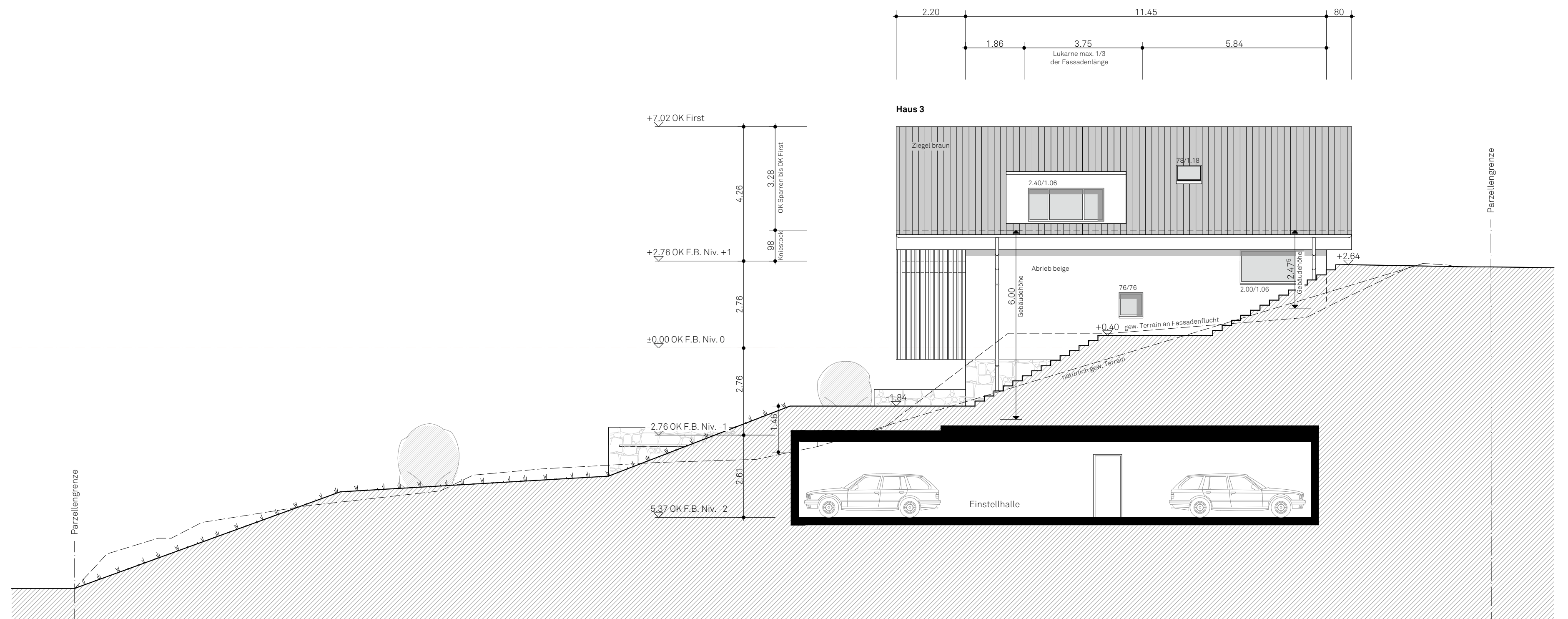
Haus 3 - Südostfassade
