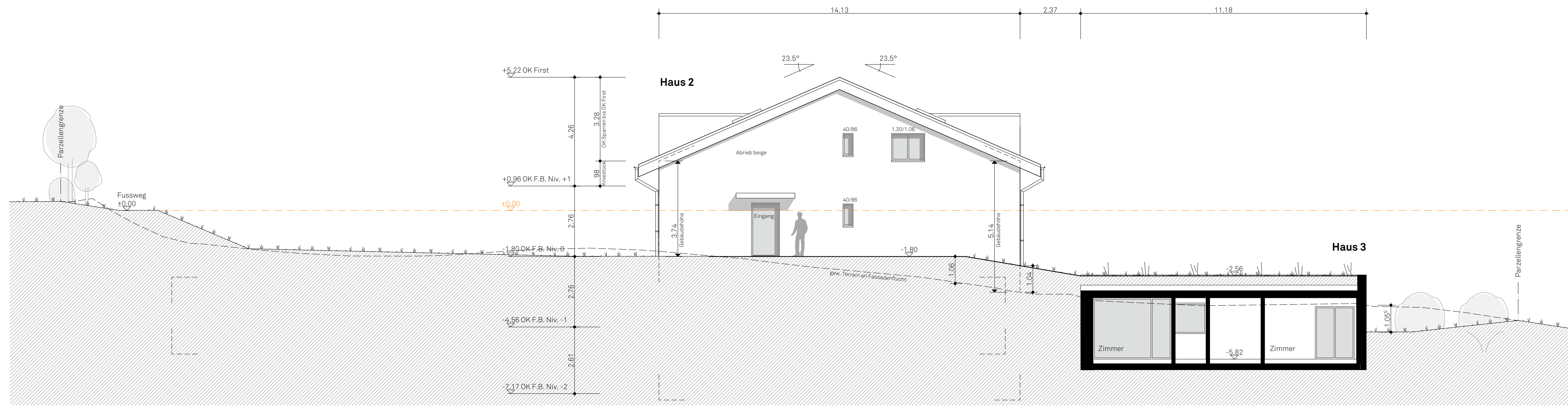
Haus 2 - Nordfassade
