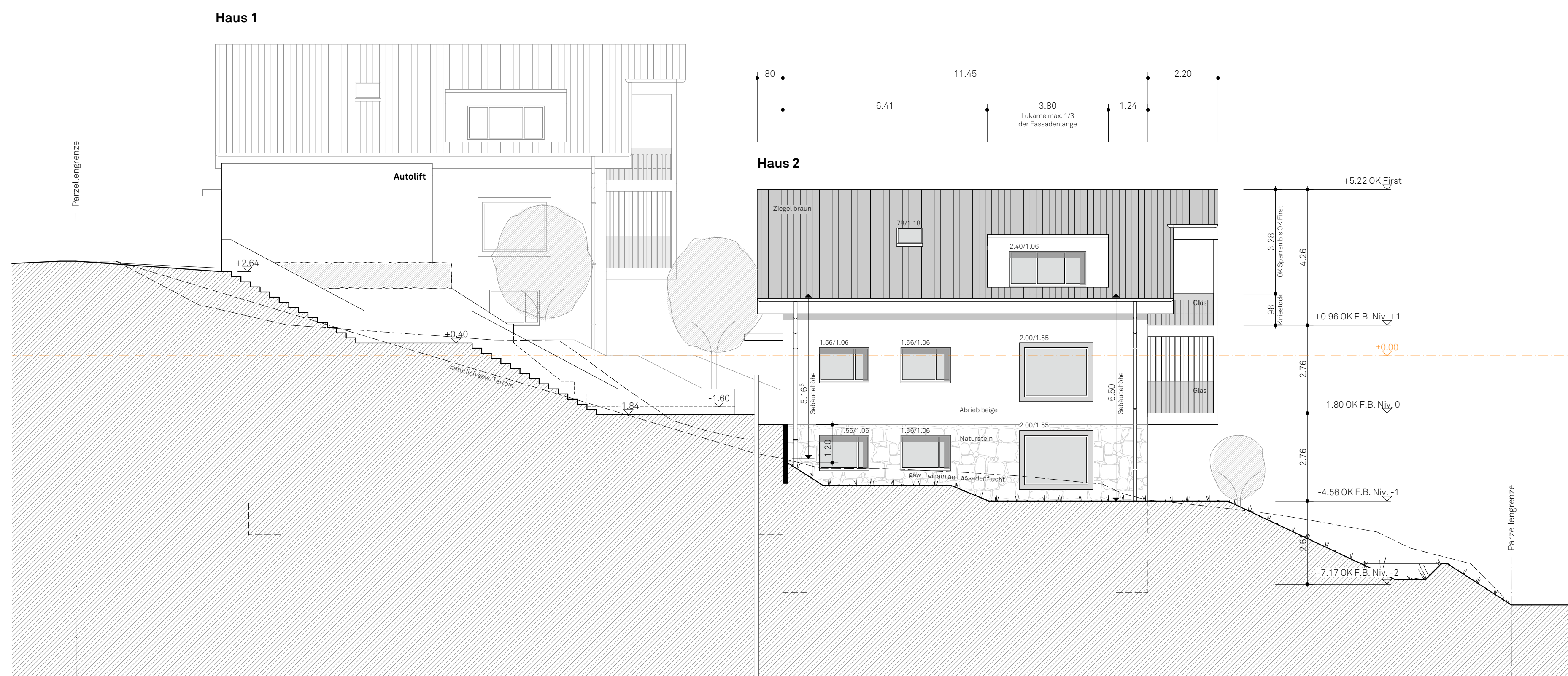
Haus 2 - Westfassade
