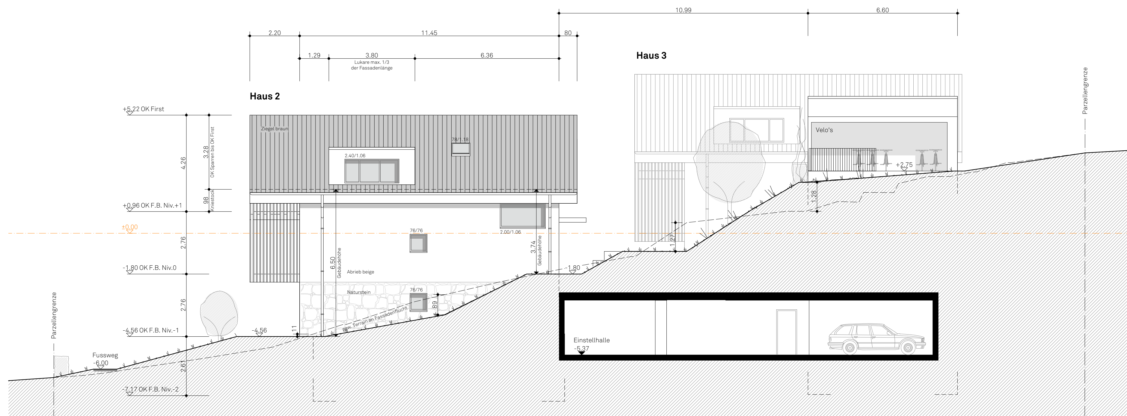
Haus 2 - Ostfassade
