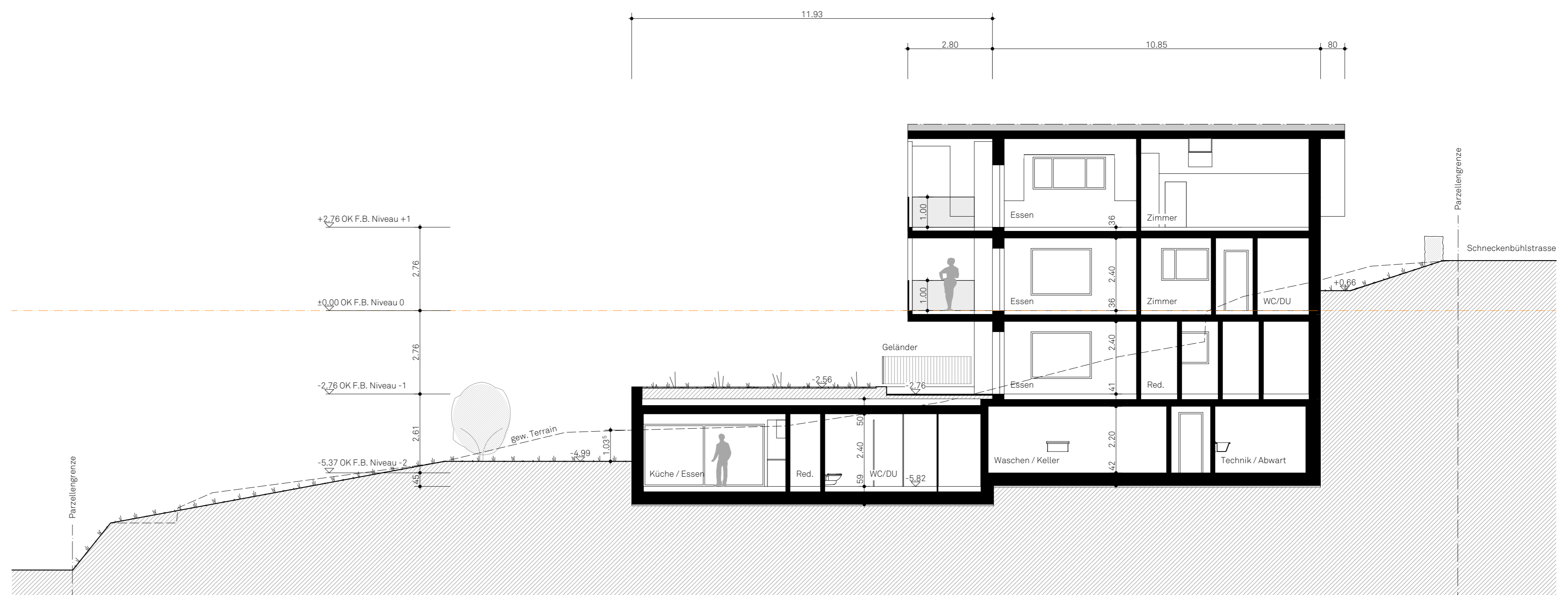
Schnitt D - Haus 3
