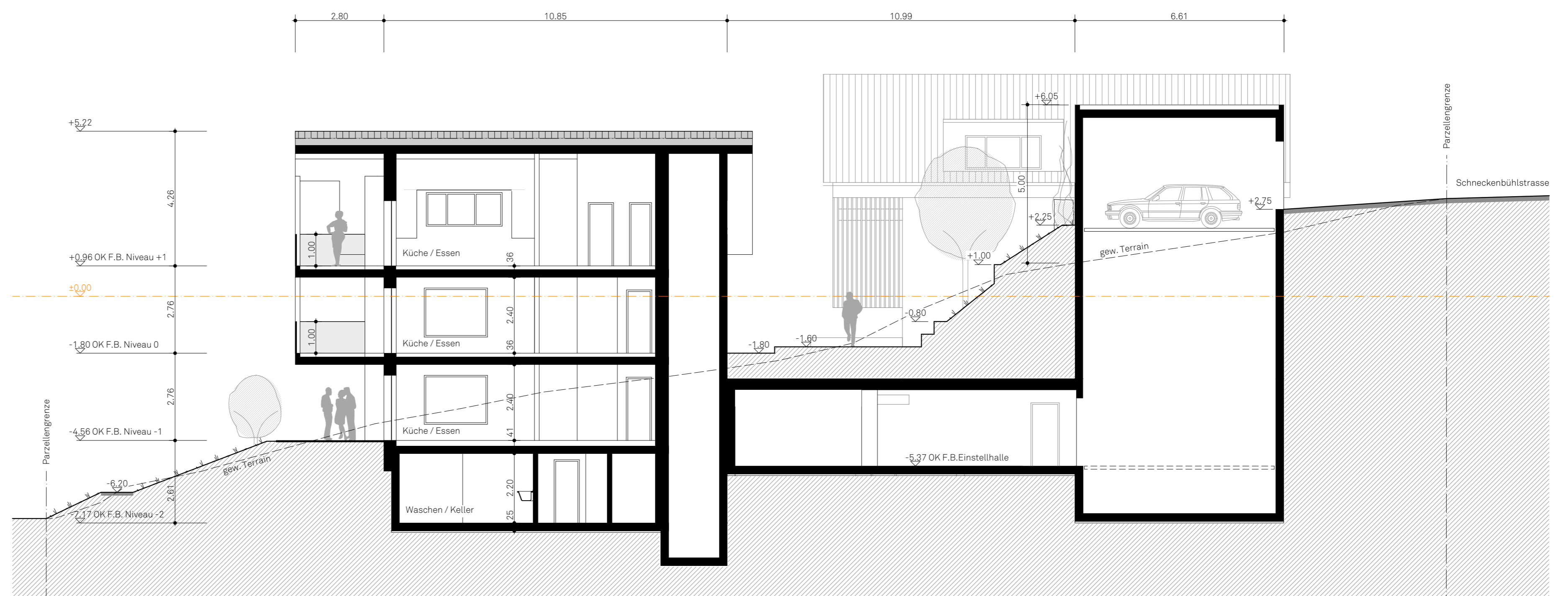
Schnitt C - Haus 2
