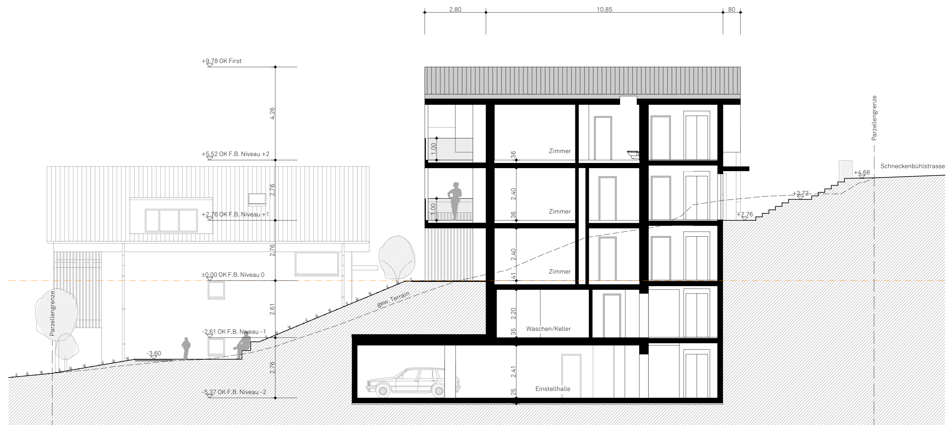
Schnitt B - Haus 1
